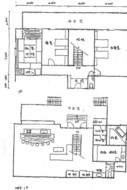
間取図
