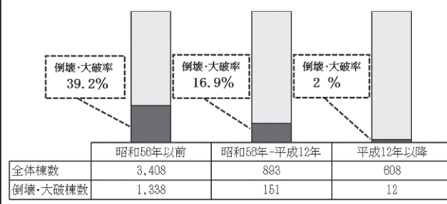
能登半島地震による倒壊・大破した木造家屋
