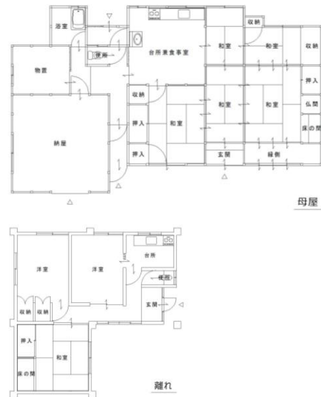
間取図
