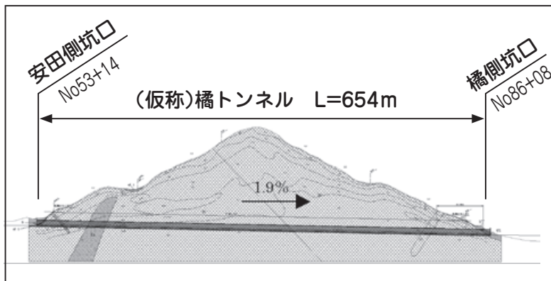
(トンネル部縦断面図)
