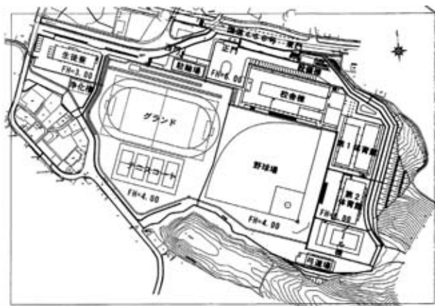
統合高校の平面図
